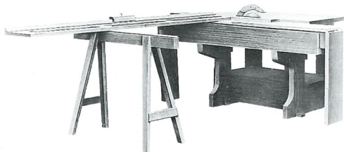
Eine der ersten Altendorf Formatkreissägen aus Holz. Baujahr 1906.
