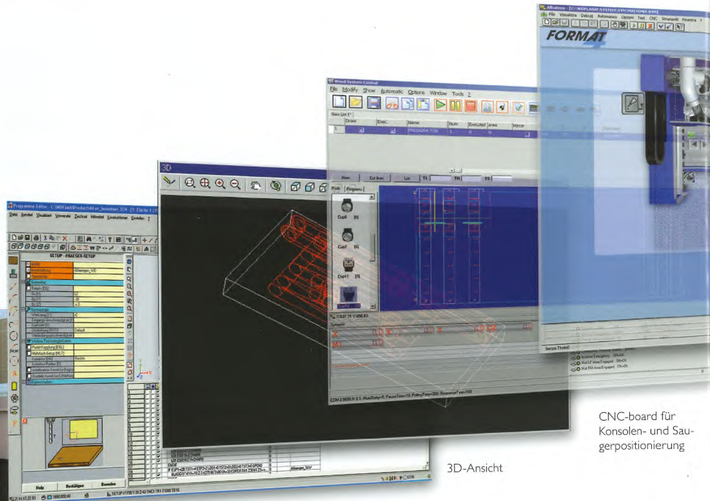
Editor Programmieroberfläche
