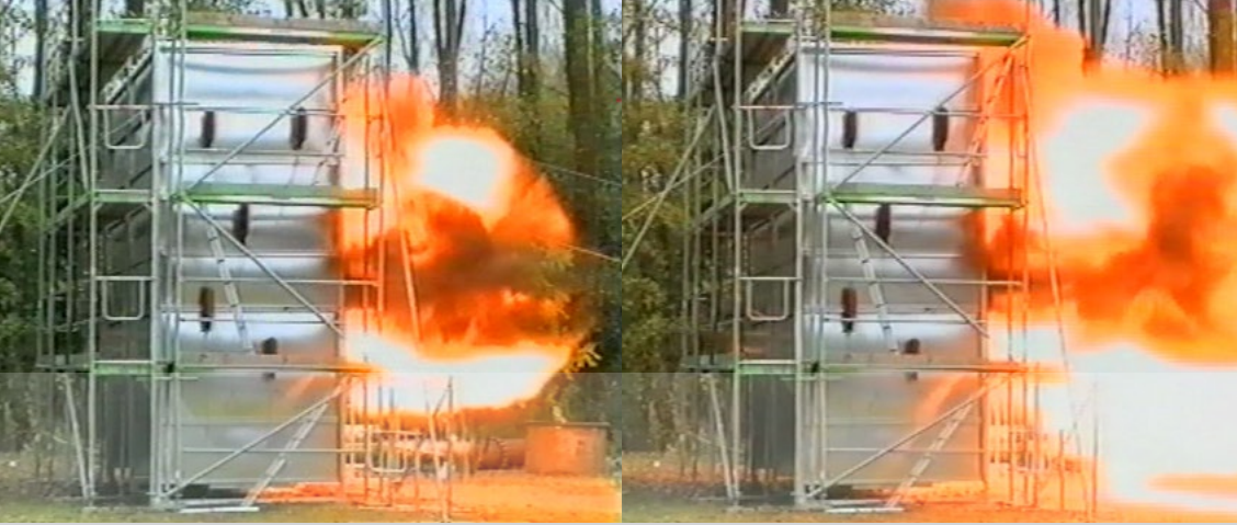
Explosionsversuch mit 220 mbar
