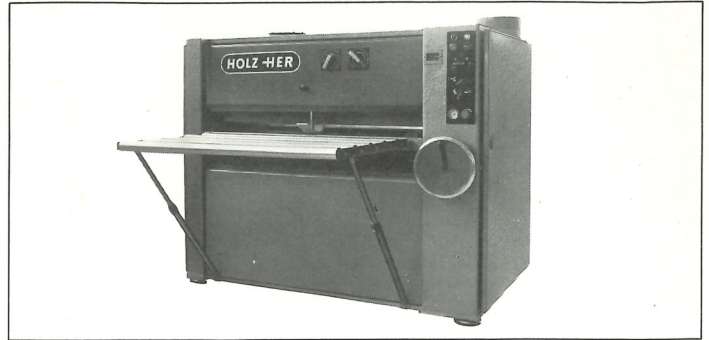
Feinschliffautomat 1370 mit Einstellautomatik Schleifbreite max. 1100 mm Durchlaßhöhe max. 100 mm Vorschubgeschwindigkeiten 7, 11, 15, 20 m/min Bandgeschwindigkeit 13 m/sec
