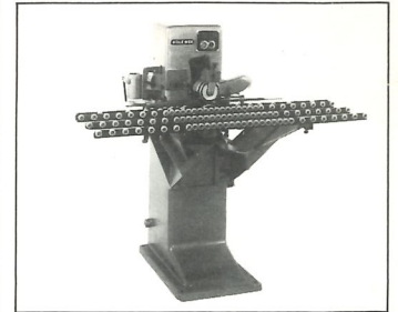
Umleimerfräse 1362 Durchlaßhöhe 15 – 70 mm Motorleistung 2,2 kW
