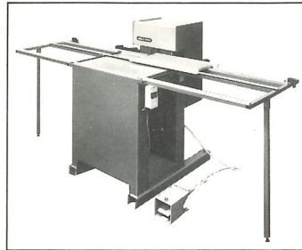
Umleimer-Kapp- und Auslinksäge 1240 max. Leistenabmessungen: 65 mm hoch, 40 mm breit Aggregat schwenkbar 5°, 15°, 22,5°, 30°, 45°, 90° Motorleistung 0,75 kW
