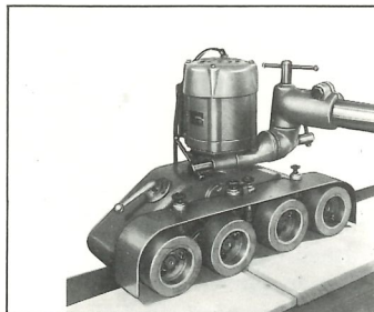
Vorschubapparat 1112 2, 4, 5, 6, 10, 12, 15, 30 m/min Motorleistung 0,55/0,75 kW Vorschubrollen-Ø 110 x 50 mm mit Universalständer
