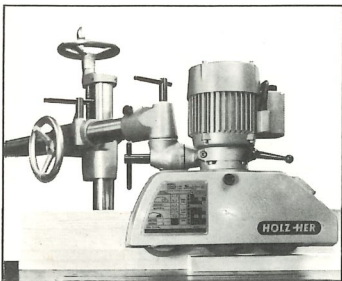
Vorschubapparat 1117 4, 6, 8, 10, 12, 15, 20, 30 m/min Motorleistung 0,55/0,75 kW Vorschubrollen-Ø 110 x 50 mm mit Universalständer
