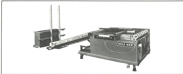
Stapelautomat 1110 Werkstückmaße: Länge 400 – 2500 mm, Breite 140 – 1100 mm, Dicke min. 5 – max. 50 mm Einlaufhöhe 800 – 980 mm Stapelhöhe max. 1800 mm bei schweren (max. 40 kg) und glatten Werkstücken ca. 1500 mm Vorschub 17 und 34 m/min
