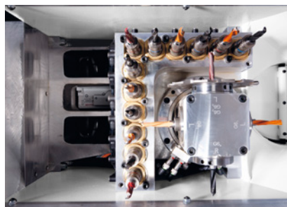
Bohrkopf V12/H4: HIGH-SPEED Bohrkopf bis 7500 1/min mit 12 Vertikalspindeln, Nutsäge und 4 Horizontalspindeln 0/90° schwenkbar. Schnelles Bohren inkl. Nuten in X/Y-Richtung.
