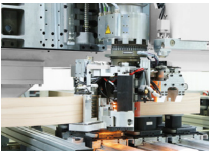
Kantenverleimung für Bauteile bis 100mm Höhe
