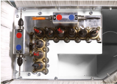
Bohrkopf V9/H4: HIGH-SPEED Bohrkopf bis 7500 1/min mit 9 Vertikalspindeln und 4 Horizontalspindeln.
