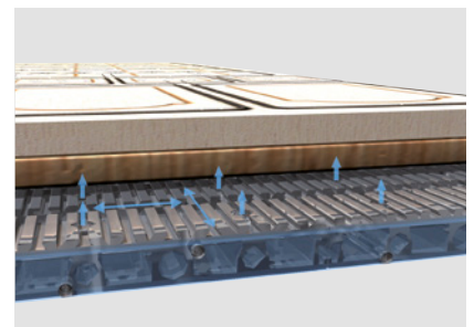
Vakuum-Rastertisch mit Luftkissenfunktion: Die Übertragung des Vakuums ist in die Konstruktion des Aluminiumrastertisches integriert. Durch die Luftkissenfunktion fällt das Handling großformatiger plattenförmiger Werkstücke leicht.
