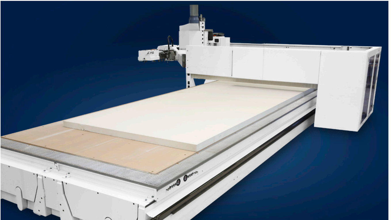
Maschinentiefe XXXL: Bauteile bis über 3 000 mm Breite für die Plattenbearbeitung für Bauelemente.
