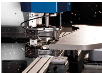
Perfektes Kantenfinish durch getastetes Kombi-Bündigfräs-/ Nachputzaggreat
