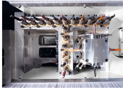
Bohrkopf V17/H4: HIGH-SPEED Bohrkopf bis 7500 1/min mit 17 Vertikalspindeln, Nutsäge und 4 Horizontalspindeln 0/90° schwenkbar. Weniger Bohrtakte inkl. Nuten in X/Y-Richtung.
