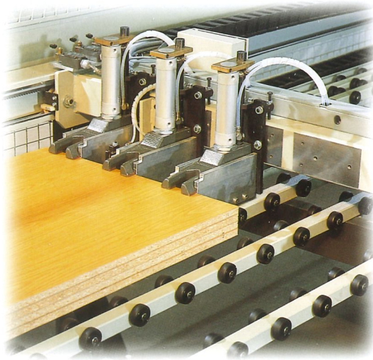
Paketklemmer in Doppelfingerausführung
