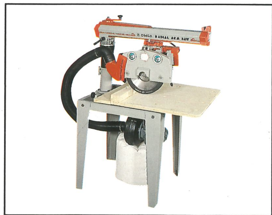
Cod. 725443000 GRUPPO ASPIRATORE DUST EXTRACTION UNIT ABSAUGVORRICHTUNG GROUPE D'ASPIRATION AFZUIGINRICHTIG GRUPO DE ASPIRACION RN 700 - 600 - 450
