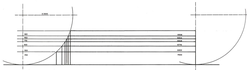
Diagramma capacità di taglio - Cutting capacity diagram - Schnittkapazität - Diagramme de coupe Zaagdiagrammen - Diagrama de capacidad de corte
