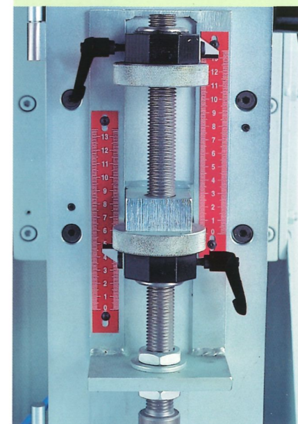
Einstellung der beiden Bohrebenen
