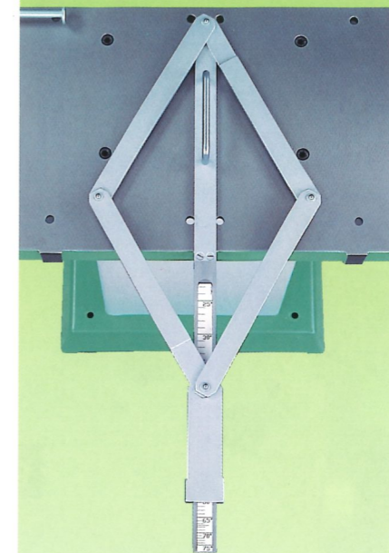
Doppelwinkelverstellanschlag mit Einstellbereich 22,5° bis 75° (Sonderzubehör)
