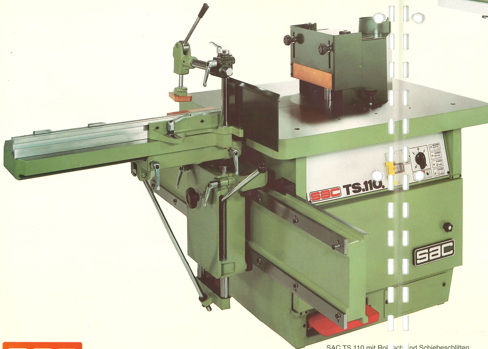
SAC TS 110 mit Rolltisch und Schiebeschlitten.
