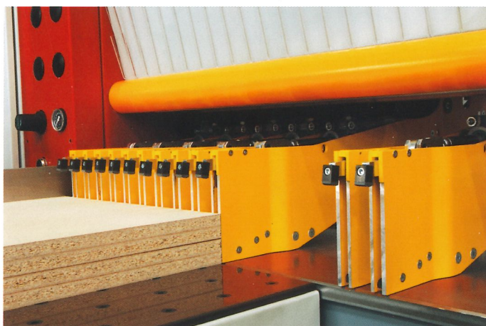
Abschieben und Ausschieben mit dem Grip-Push Klemmer ERGONOMIE PLUS+
