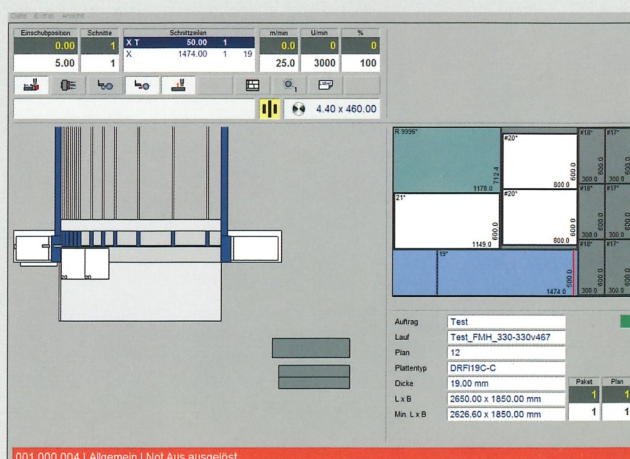
MCS Evolution - „Výrobná strana“ Roviny rezu sa dajú simulovať a optimalizovať na ovládacom pulte.
