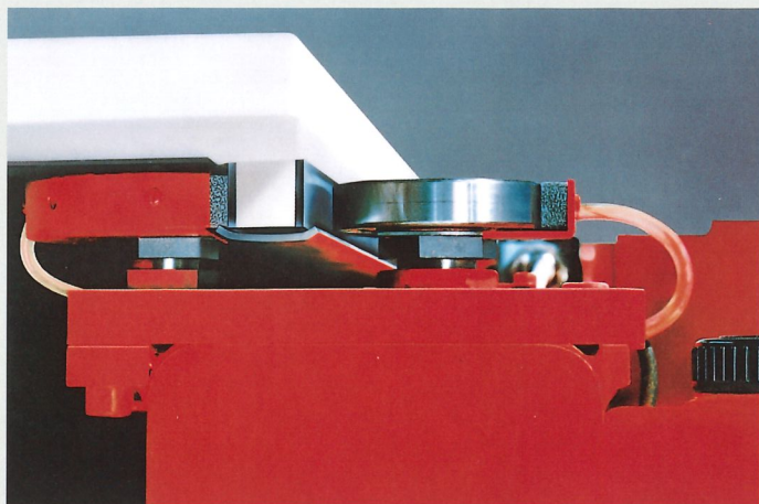
Vysokovýkonné plošné vedenie - najvyššia presnosť
