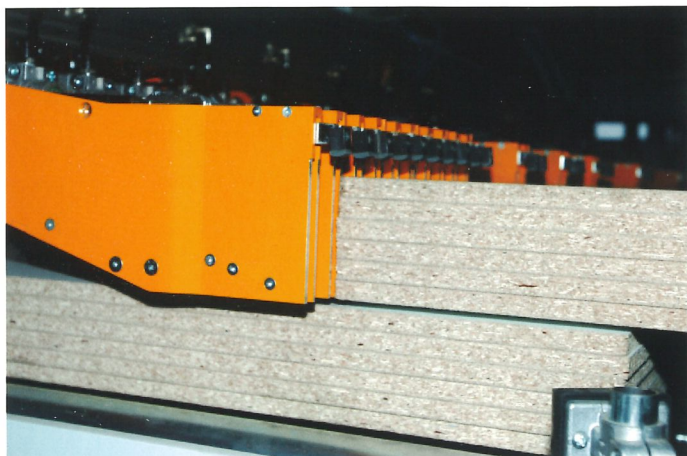
Strihové svorky - posúvanie so svorkami
