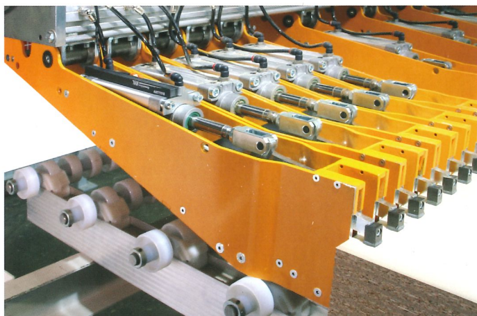
Strihová svorka - voliteľne integrované meranie hrúbky balíka
