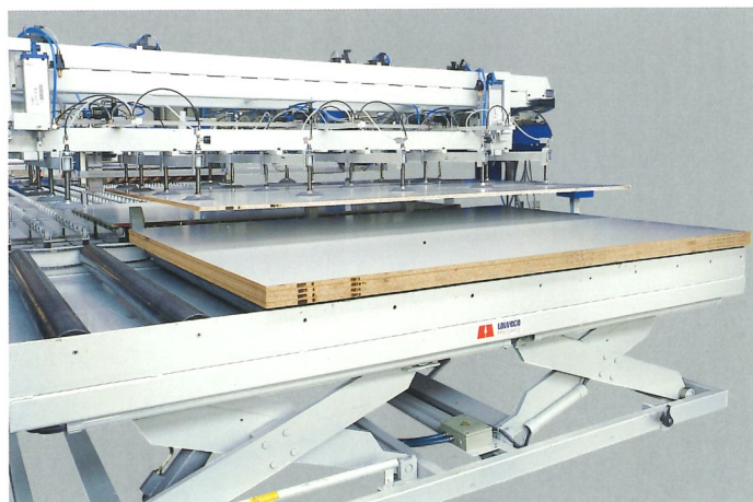
Vákuové podávanie - doprava citlivých dosiek
