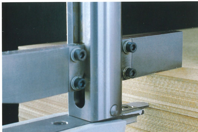
Posúvanie tenkých dosiek - podávanie s presnosťou na kus
