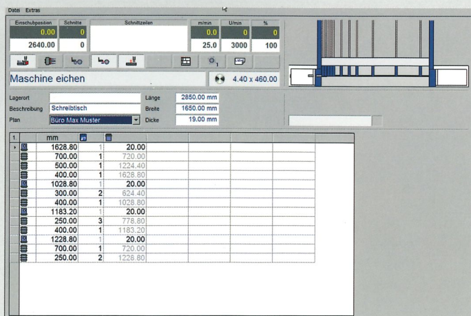
MCS Evolution - „Ručná strana“ jednoduchá a rýchla obsluha
