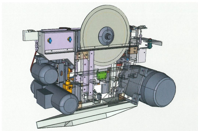
Agregát píly Evolution - najvyšší výkon rezania
