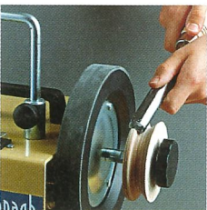
la 100 Profilierte Lederabziehscheibe für Innenflächen von Hohleisen und Geißfüßen
