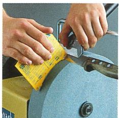
wm 100 Winkellehre zum Einstellen und Messen des Schleifwinkels
