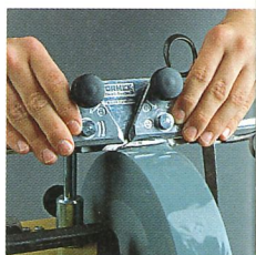
svx 150 Vorrichtung für alle Scheren, auch Heckenscheren
