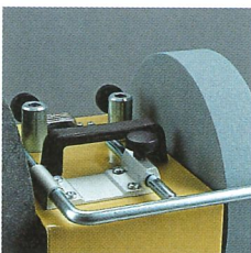
xb 100 Horizontalhalter für die Universalstütze
