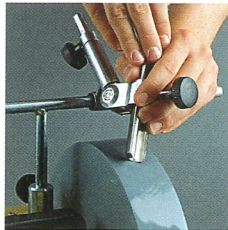
svd 180 Vorrichtung für Drehröhren und Schnitzhohleisen
