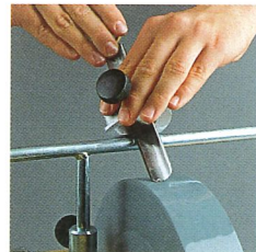
svs 40 Vorrichtung für Geißfüße bis 40 mm Breite
