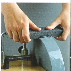
sp 650 Steinpräparierer, reguliert die Körnung des Schleifsteins
