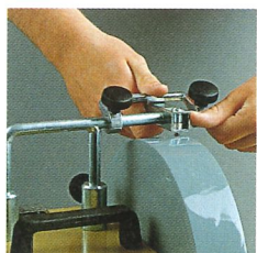
adv 50 d Abdrehrvorrichtung, macht den Stein kreisrund und plan
