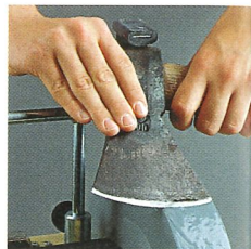
sva 170 Vorrichtung für Beile und Äxte bis 170 mm Höhe
