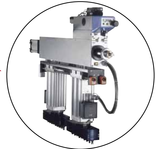
Gruppo forante verticale con guide a ricircolazione di sfere e lettura elettronica dello spostamento. Vertical boring group with ball bushing guides and electronic digital readouts. Bohrereinheit mit Kugelführungselementen und digitaler elektronischer Anzeige. Tete avec coulisses a billes et lecteur digital electronique. Cabezal con guias a recircolacion de esferas y indicador digital electronico. Вертикальная сверлильная группа на направляющих шариковых втулках и электронные цифровые счётчики.
