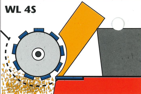
Rotor-Ø 368 mm, grand rotor et angle de coupe importante permettent un gros débit surtout avec des matériaux à broyer en forme de panneaux.
