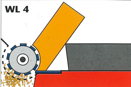
Rotor-Ø 252 mm, avec un grand couple.
