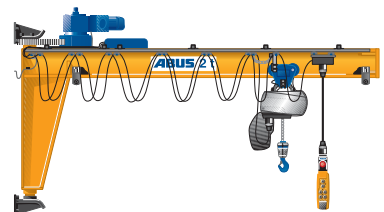
Abb.: VW mit Zusatzausstattungen (elektrisches Schwenkwerk und verfahrbare Steuerung)
