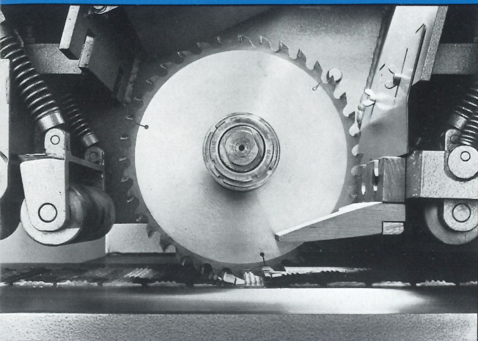
Sägepaket mit durchtauchender Transportkette in Zwangsführung. Eingesetzter halber Druckschuh für kurze Werkstücke.
