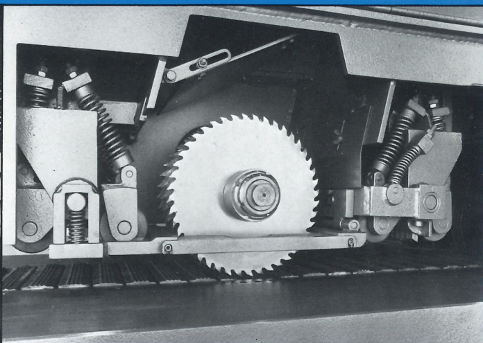
Sägepaket mit 5 doppelt gelagerten Druckrollen und durchgehendem Druckschuh für extrem kurze und schmale Werkstücke.
