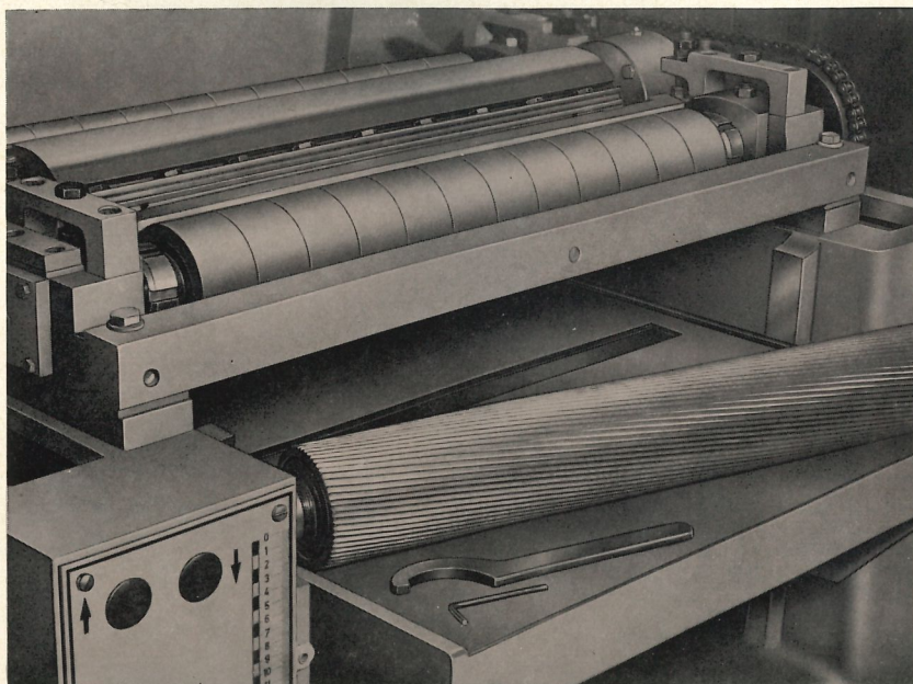
Abb. zeigt: Auswechselbare Gummisegmentwalze
