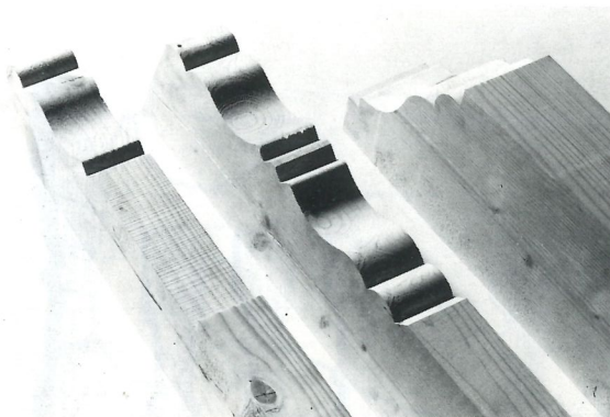
Stirnseitige Bearbeitung von Werkstücken für Dachkonstruktionen (Pergolen). Durch den festen Tisch lassen sich Werkstücke jeder Länge bearbeiten.
