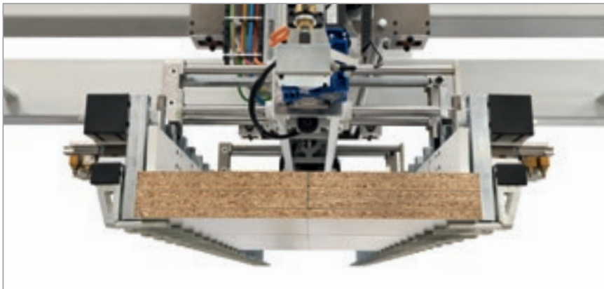
Le châssis à pinces avec presseur garantit la prise de paquets aussi bien en file simple que double.
