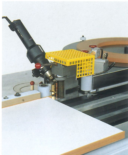
Обработка прямых кромок. Агрегат с подачей горячего воздуха для толстых кромок ПВХ (опция)
