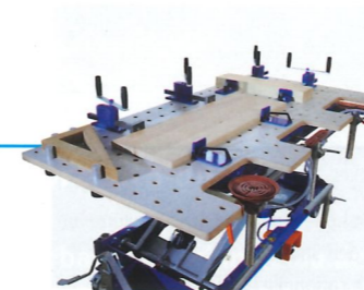
Lochplatte zum Pressen und Montieren nutzbar
