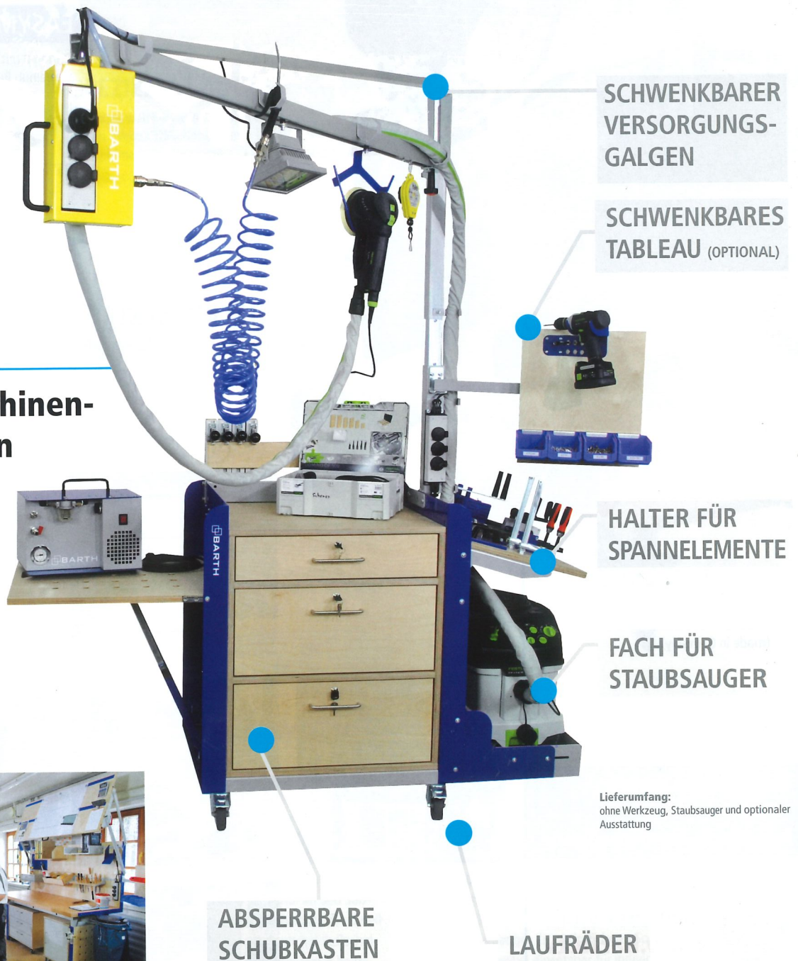
Das orgaCAR im Einsatz!
