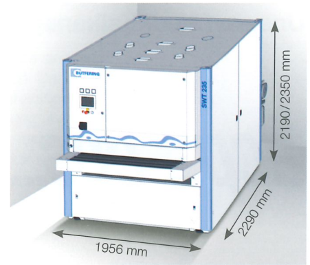
Maße der SWT 235
