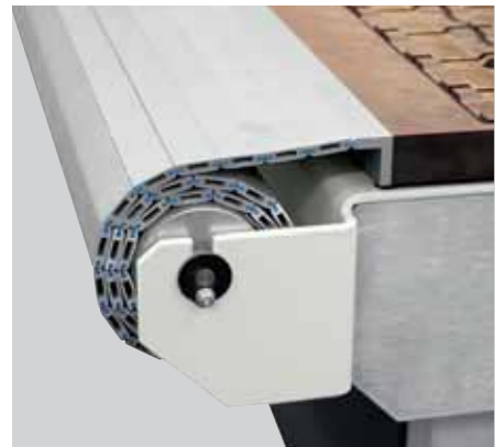
Roller shutter intrusion detection device (optional) Dispositif anti-intrusion enroulable (option) Vorrichtung gegen Eindringung. (Sonderzubehör)
