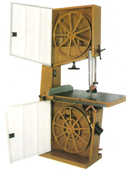
Compact S mit Guß-Speichenrädern
