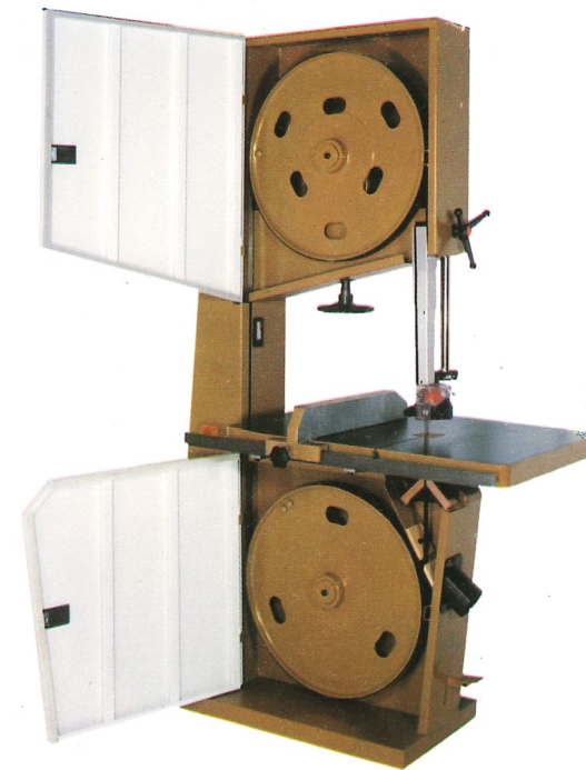
Compact C mit Guß-Scheibenrädern
