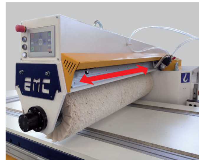
Sistema automatico di spruzzo della pasta Automatic system for abrasive wax application Système automatique pour application de la pâte abrasive
