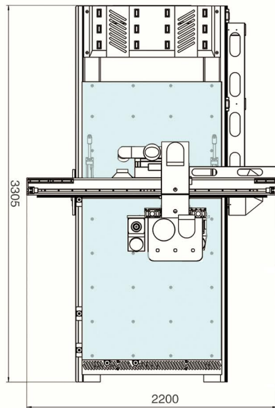
E2-9 NESTING
