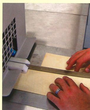
automatyczne podawanie forniru po ręcznym ustawieniu
