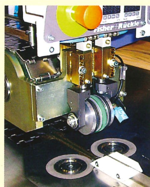
sprawdzone podawanie z tarczami
