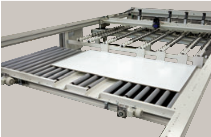
Tavolo elevatore di carico Loading lift table Table élévatrice de chargement
