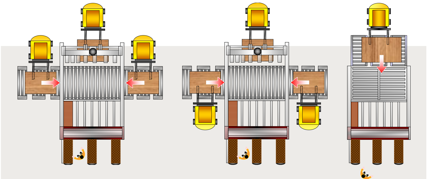
Rullive di precarico L'utilizzo di una o più rullive di precarico favorisce la continuità lavorativa della sezionatrice. Soluzioni di carico della pila completa e scarico della pila incompleta offrono adeguate risposte alle esigenze di spazio e produttività.
