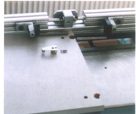
▲ Schrankverbindungsbeschläge
