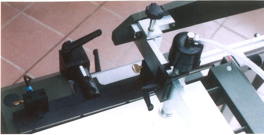
▲ Pneumatischer Anschlagkamm mit Winkelfehler-Ausgleichssystem
