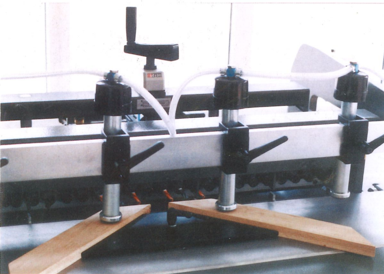
▲ Gehrungsrahmen 45°
