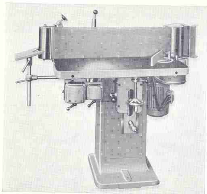
Kantenschleifmaschine FLK 4
