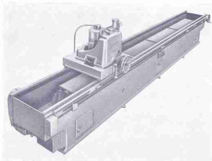
G4 Schwere Furniermesser- schleifmaschine
