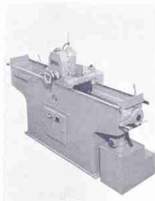
GB1 Hobelmesserschleifmaschine
