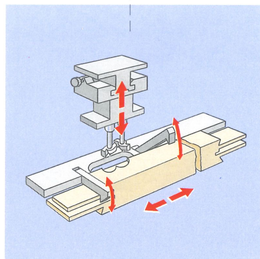
■ Bohrkopf BKF 2 – schnellwechselbar, 2 Spindeln für Ecklager-Bohren am losen Rahmenteil, komplett mit Anschlagssystem und 2 Klappanschlägen (Sonderzubehör).
