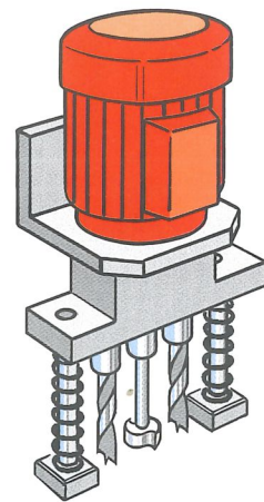
Standardbohrkopf OBM
