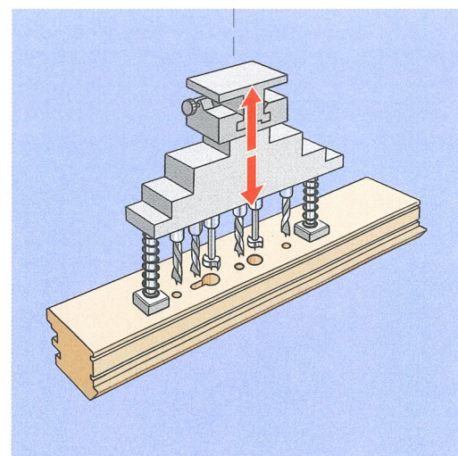
■ Bohrkopf BKF 6 – schnellwechselbar, zum Bohren der Türschutzgarnitur – komplett mit Anschlag, Entspäne- und Folgesteuerung der Grundmaschine.
