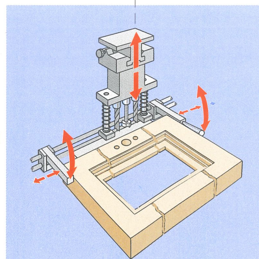
■ Anschlagssystem für mittiges Bohren im Fensterflügel. (Sonderzubehör)
