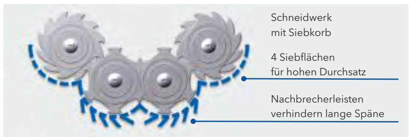
Schneidwerk (Schema)
