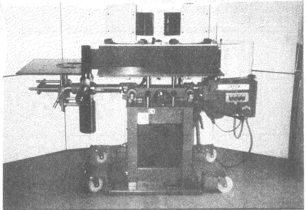
BSM 2000 Kantenschleifmaschine mit aufgeklappter Furnier- kantenschleifeinrichtung
