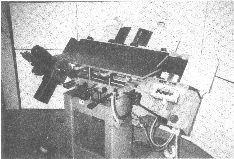
Gesamtes Schleifaggregat (45° geschwenkt) mit aufgeklappter Furnier- kantenschleifeinrichtung
