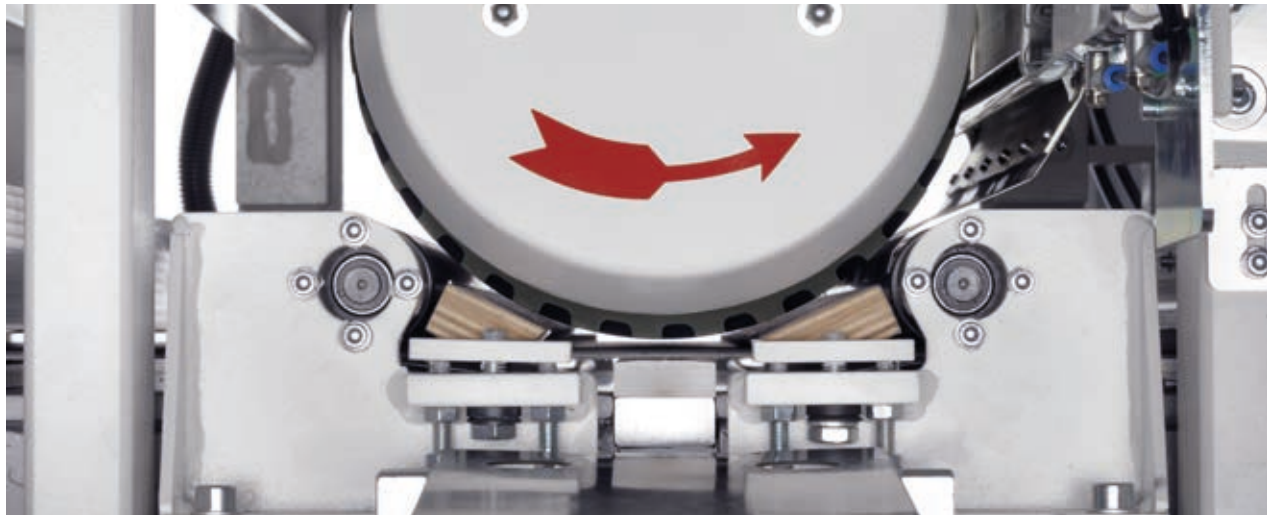
Gummibeschichtetes Schleifwalzenaggregat
