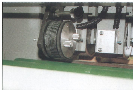
Signiereinrichtung zur Lamellenkennzeichnung
