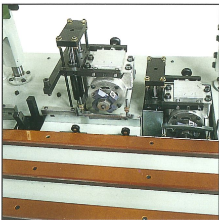
Refilatori copiatori con regolazioni dall'esterno Affleureuses copieurs avec réglages de l'extérieur Kopierbuendigfraeseaggregat mit aeusserer Regulierung
