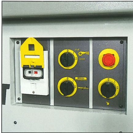
Quadro comandi elettrici Tableau commandes électriques Zentralisiertes elektrisches Steuerpult
