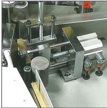
Intestatori pneumatici (cesoia) anteriore e posteriore Coupes en bout pneumatiques (cisaille) à l'avant et à l'arrière Vorderes u. hinteres pneumatisch gesteuertes Abkappaggregat
