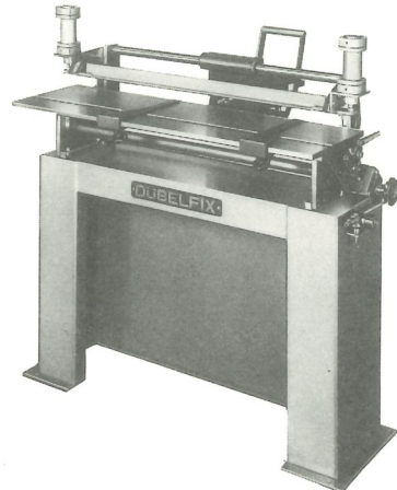
DB 1-U (horizontale Arbeitsstellung)
