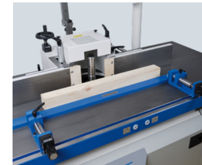
Gegenanschlag
