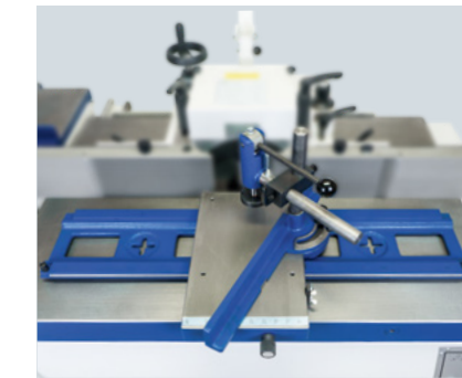
Schiebeschlitten
