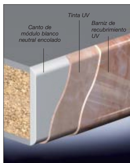
Composición de capas del método print line
