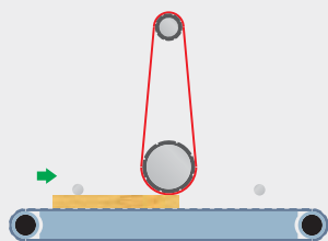
I BROUSÍČÍ JEDNOTKA TYPU R BROUSÍČÍ VÁLEC – OCELOVÝ Ø 120 MM
