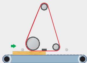
I BROUSÍČÍ JEDNOTKA TYPU C BROUSÍČÍ VÁLEC + PEVNÁ MECHANICKY NASTAVITELNÁ PATKA
