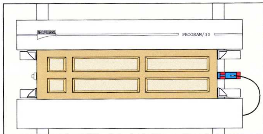
Cilindri ausiliari orizzontali per telai con montante centrale.
