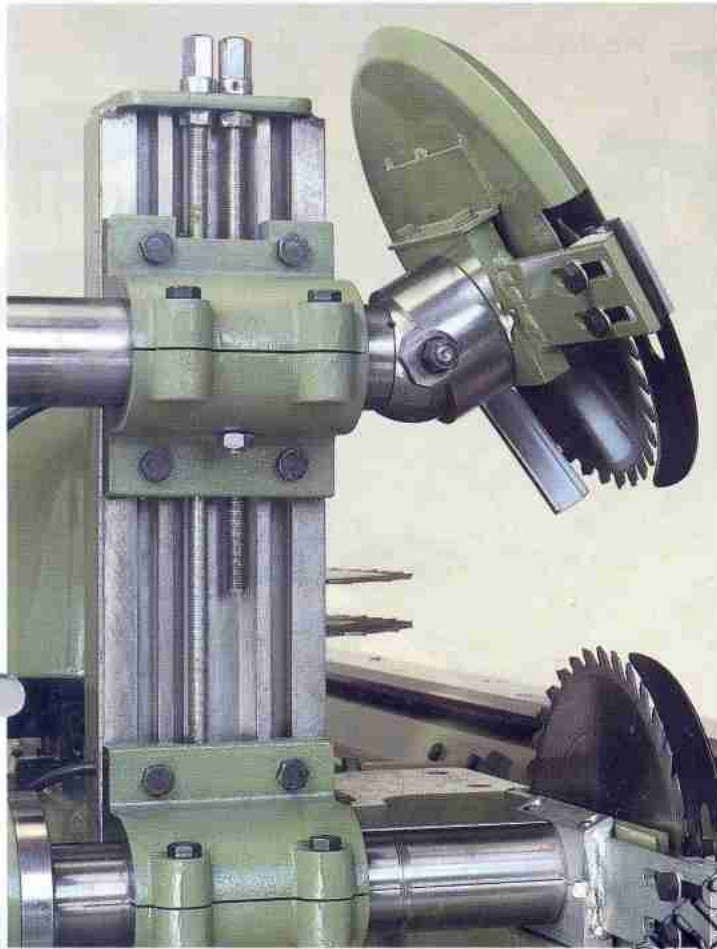
Handrad Klemmgriff Skala Klemmhebel Handgriff
