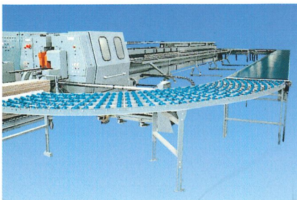
ZHR 10 an einer eineinhalbseitigen Kantenanleimmaschine
