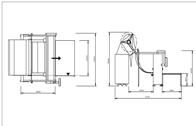
Layoutbeispiel: VKS200 mit Haspelzuführung
