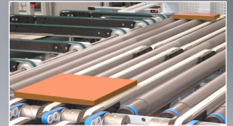
Geteilte Querriemen in der Rollenbahn
