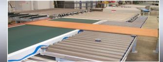
Geteilte Querriemen in der Rollenbahn
