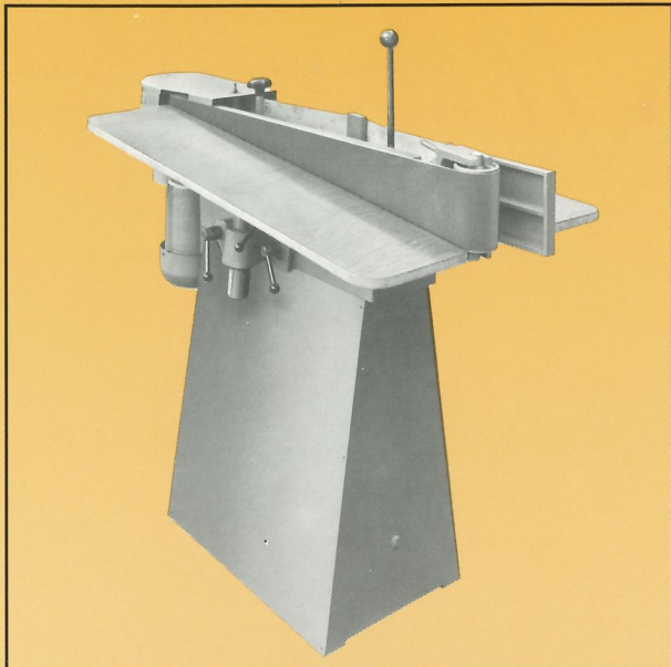
KSM 1 mit leichtem Ständer
