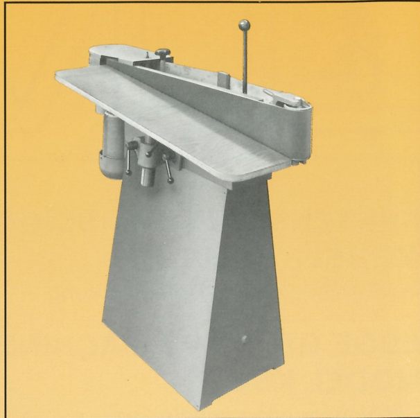
KSM 2 – ohne Furnierkantenschleifeinrichtung
