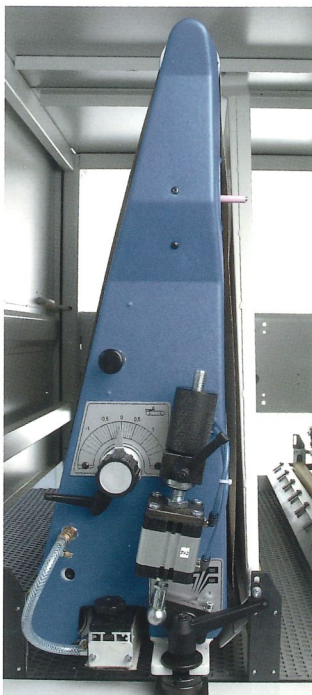
Kombiniertes Aggregat/ Schleifwalze/starrer Schleifschuh Luftkissen-Schleifschuh
