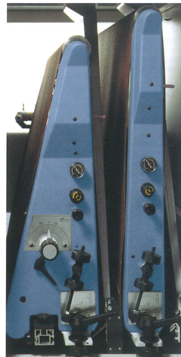
2 Aggregate: 1. Kalibrieraggregat und 2. Kombiaggregat Schleifwalze / starrer Schleifschuh
