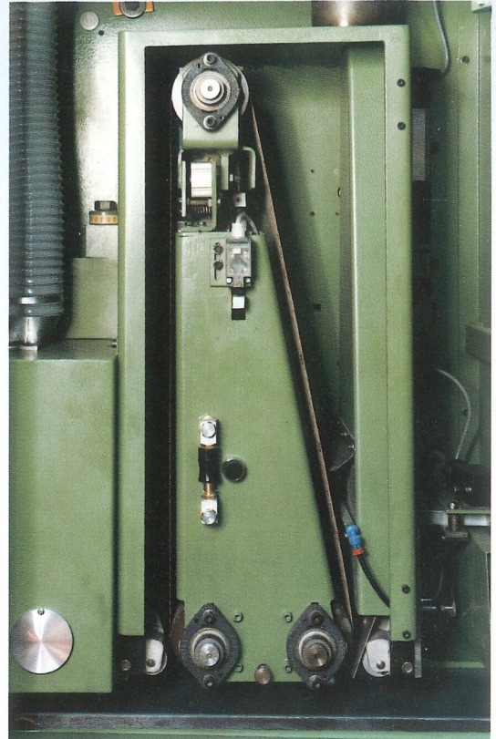
Abb./III. 3 Sanding unit Schleifeinheit Agrégat de ponçage
