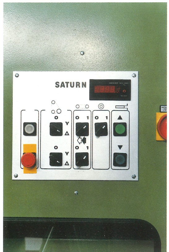
Abb./ III. 4 Control panel with digital display Bedientafel mit Digitalanzeige Tableau de commande avec lecture digitale
