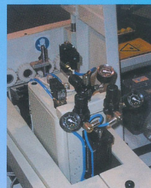
LEVIGATORE INCLINABILE Levigatura dei bordi diritti o sagomati mediante nastro abrasivo oscillante
