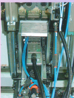
ARROTONDATORE Arrotondatura inferiore del bordo applicato a pannelli post-formati
