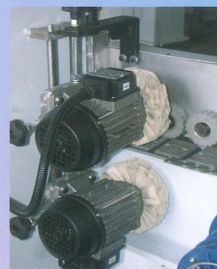
GRUPPO SPAZZOLE OSCILLANTI Perfetta lucidatura dei bordi in PVC e ABS
