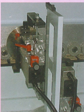
GRUPPO RIFILATORE - SPIGOLATORE Rifilatura superiore e inferiore del bordo applicato
