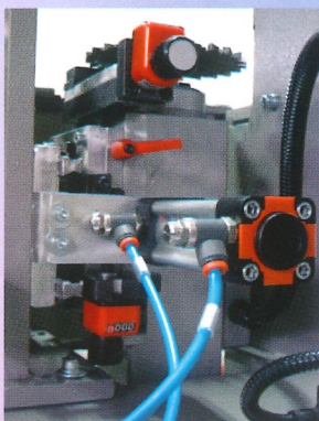
TOUPIE 0° - 90° Fresatura passante sul lato bordato o sulla parte inferiore del pannello
